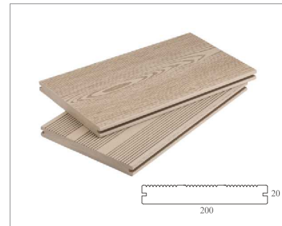
MD-200×20K 5.1kg/m
