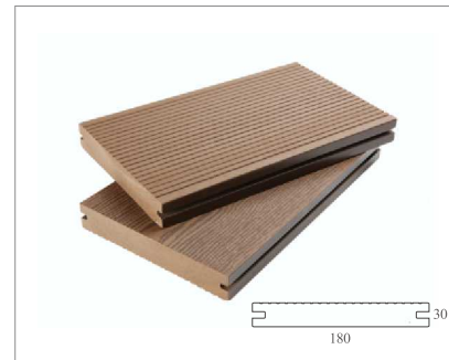
MD-180×30 7.1kg/m
