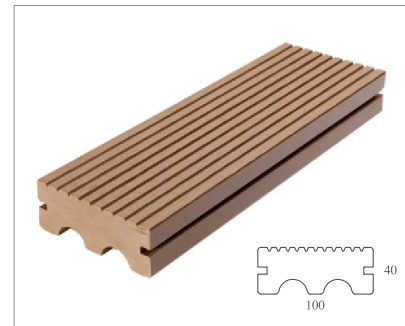
MD-100×40
