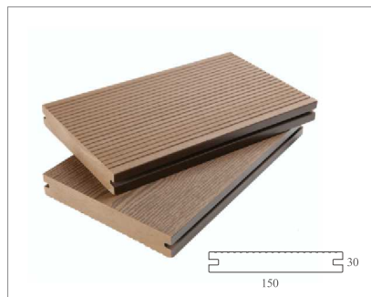
MD-150×30 5.8kg/m
