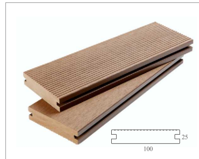
MD-100×25C
