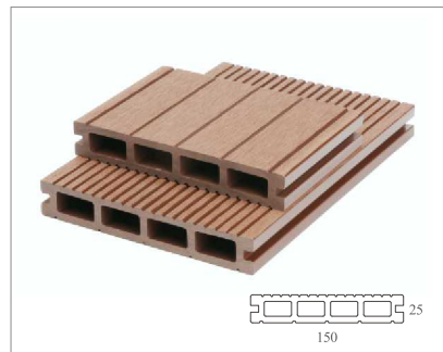
MD-150×25H 2.5kg/m
